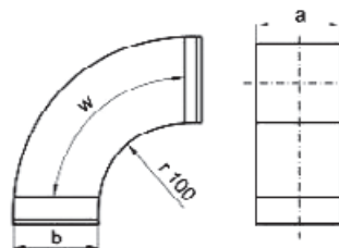
kolano symetryczne symmetrical bend
