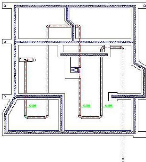
Rys.2 Przykładowy wymiennik gruntowy zlokalizowany pod budynkiem - rura PVC-U O 200/3,9; L = 48,3 m.
