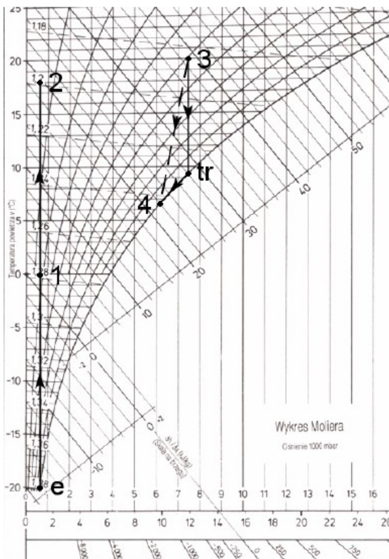
Rys.4 Przemiany powietrza na wykresie i-x w zimie: e-1 ogrzewanie powietrza nawiewanego w wymienniku gruntowym, 1-2 ogrzewanie powietrza nawiewanego w rekuperatorze, 3-4 chłodzenie powietrza wywiewanego w rekuperatorze.
